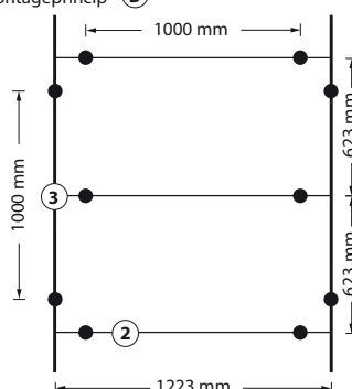
Montageprincip (B)
