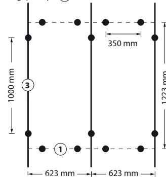
Montageprincip C
