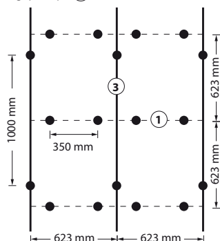
Montageprincip A
