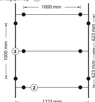
Montageprincip B
