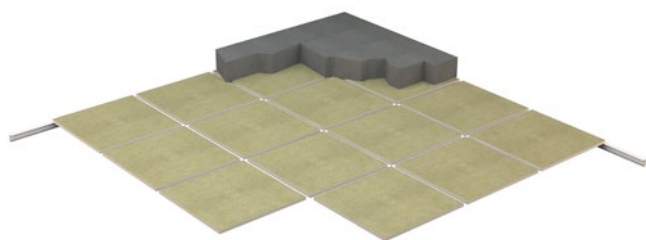
Översikt Rockfon System A Adhesive.
