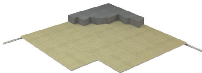
Översikt Rockfon System B Adhesive.
