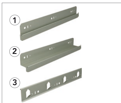
Rockfon har två montageset som ger en distans från skivan till väggen på 15 eller 65 mm. Båda seten innehåller profiler för väggmontage.
